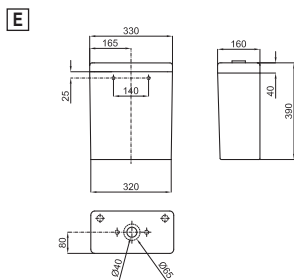
Унитаз напольный с вертикальным выходом и с креплениями 100041212 - N420150000. Включает также крепления 100077249 - N499816855. (1)
